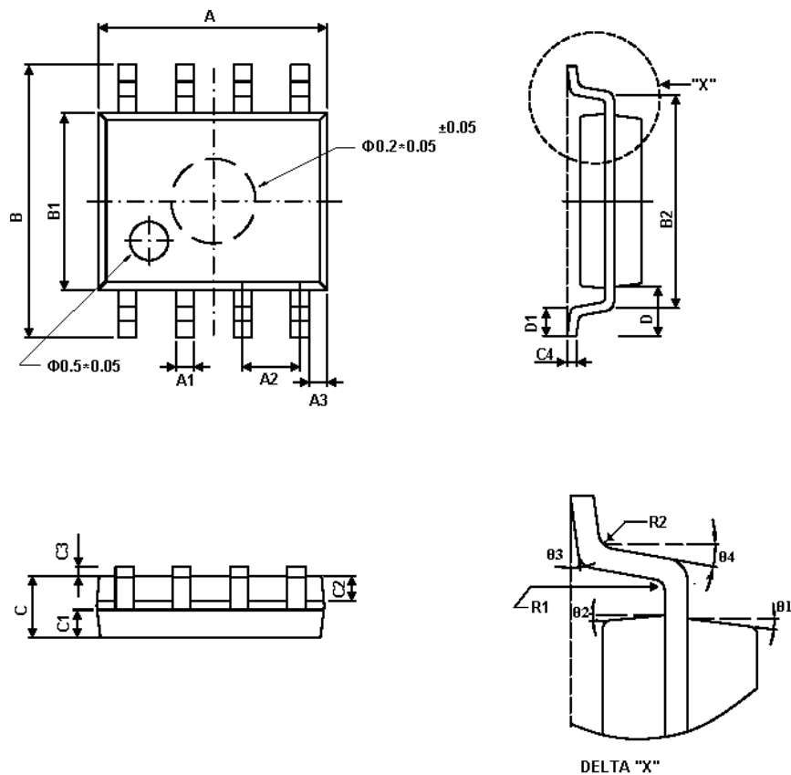
图 5 HLW8032 封装尺寸图
